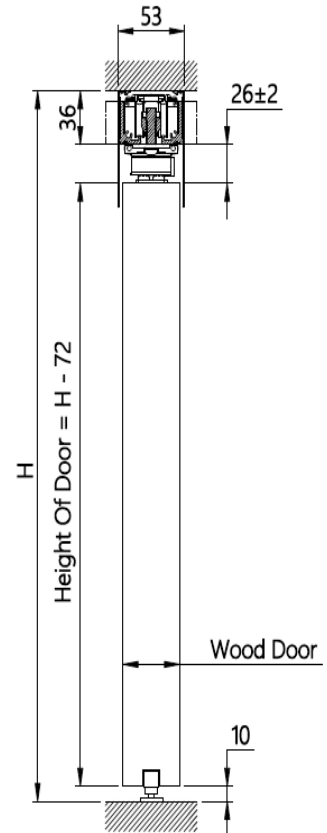
Type 3: Wooden/Aluminum Door (Bracket SDS-090-b2)
