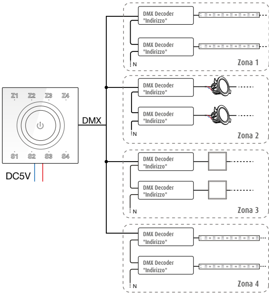
DMX DIAGRAMM
